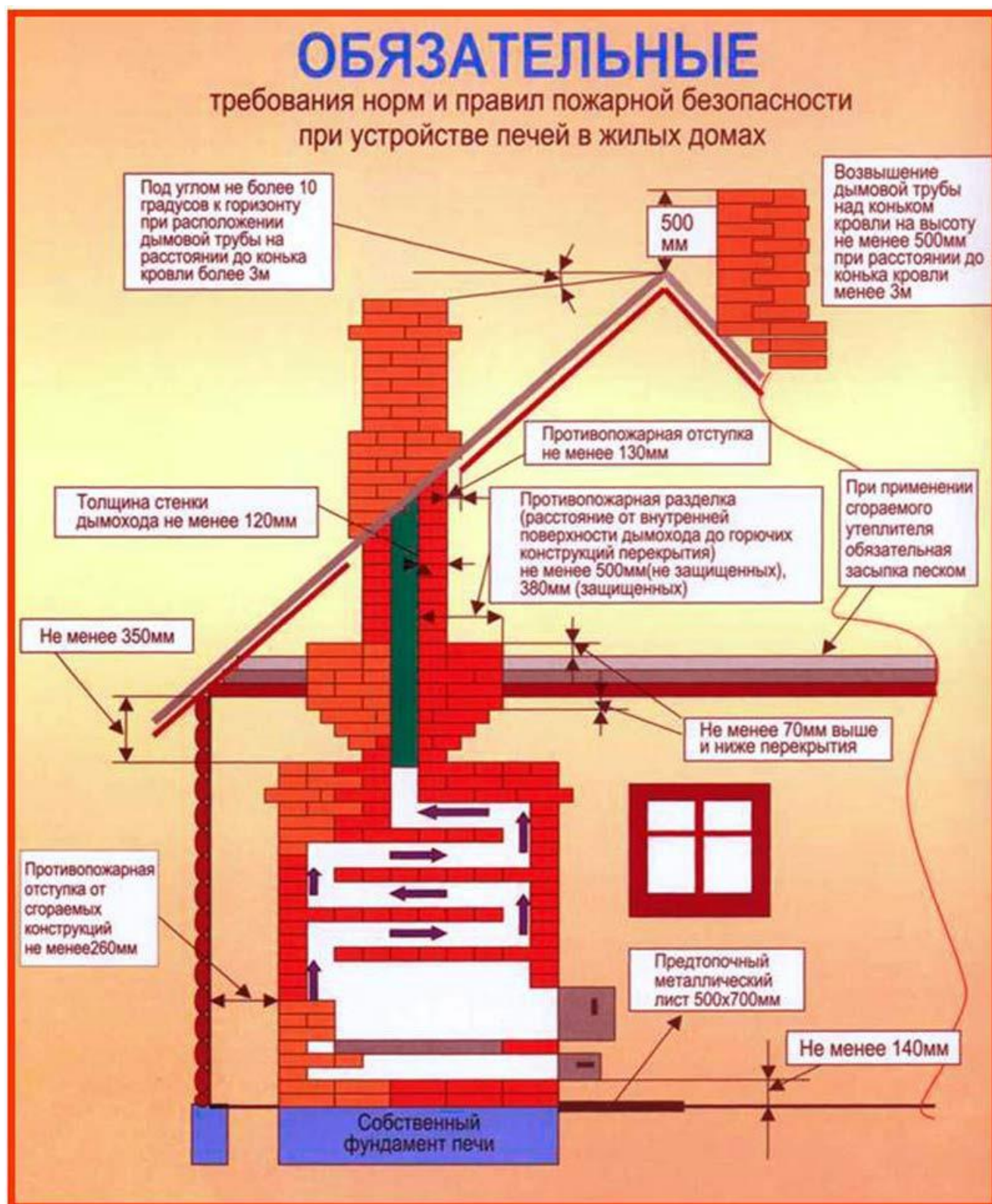
Схема противопожарных требований.
